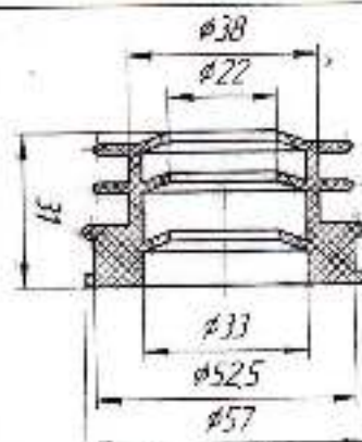
Манжета переходная D 50x25 трех лепестковая
